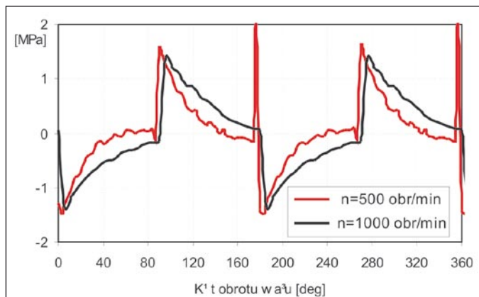
Rys. 7. Wpływ prędkości obrotowej na przebieg zmian ciśnienia w komorze cylindrowej pompy PWKZ-78 bez kompensacji
