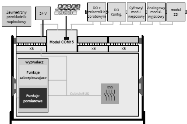
Rys. 3. Przykład rozbudowanego rozwiązania wewnątrz i zewnętrznej magistrali danych wyłącznika IZM [7]
