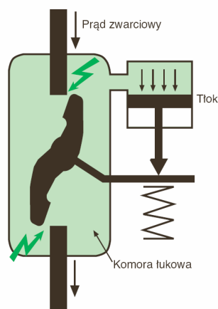
Rys. 5. Zasada dynamicznego gaszenia łuku [10]
