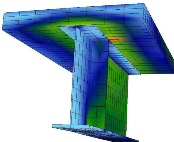
Rys. 10. . Wizualizacja wyteżenia w płycie nad żebrzem podporowym modelu bryłowego
