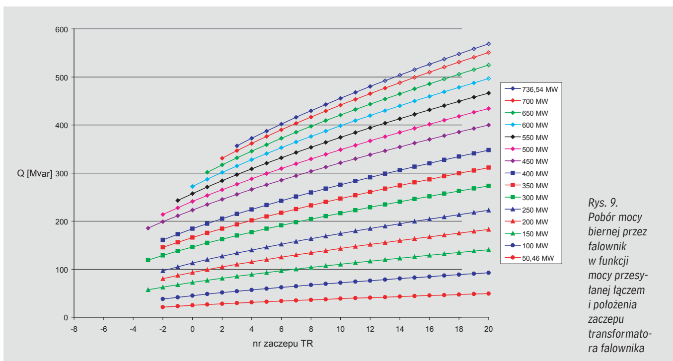
Rys. 8. Pobór mocy biernej przez prostownik w funkcji mocy przesyłanej i kąta wartości napięcia na szynach 400 kV stacji prostownikowej
