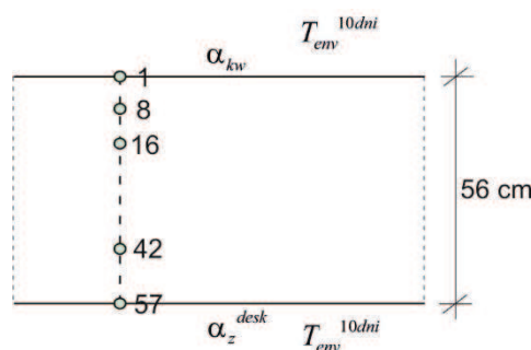
Rys. 6.37. Dyskretyzacja MRS
