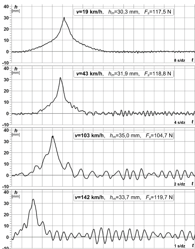
Rys. 3. Wyniki wskazujące wzrost amplitudy drgań sieci z wzrostem prędkości pociągu; naniesione wartości liczbowe oznaczają: v – prędkość pociągu, h_m – wartość maksymalną uniesienia przewodów, F_s – oszacowaną siłę statyczną
