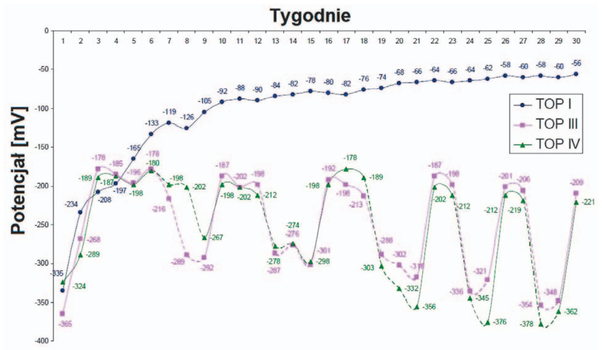
Rys. 1. Zestawienie pomierzonych potencjałów korozyjnych w czasie
