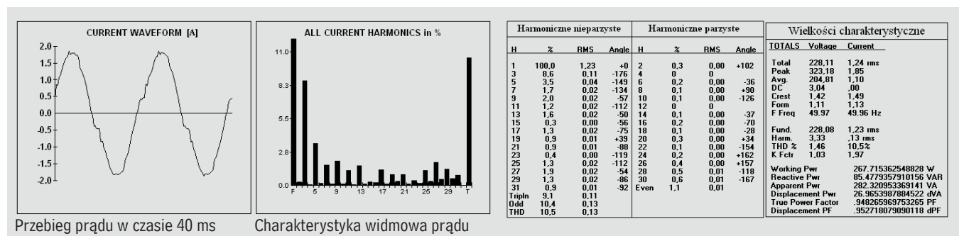
Rys. 12. Analiza prądu pobieranego przez świetłówkę liniową ze statecznikiem elektronicznym umożliwiającym regulację strumienia świetlnego. Regulator nastawiony na pośredni strumień świetlny (ze względu na zastosowaną przekładnię przetwornika pomiarowego wartości prądu i mocy należy podzielić przez 10)
