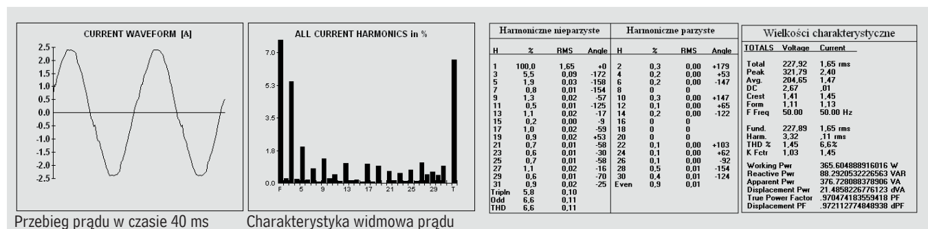
Rys. 11. Analiza prądu pobieranego przez świetłówkę liniową ze statecznikiem elektronicznym umożliwiającym regulację strumienia świetlnego. Regulator nastawiony na maksymalny strumień świetlny (ze względu na zastosowaną przekładnię przetwornika pomiarowego wartości prądu i mocy należy podzielić przez 10)
