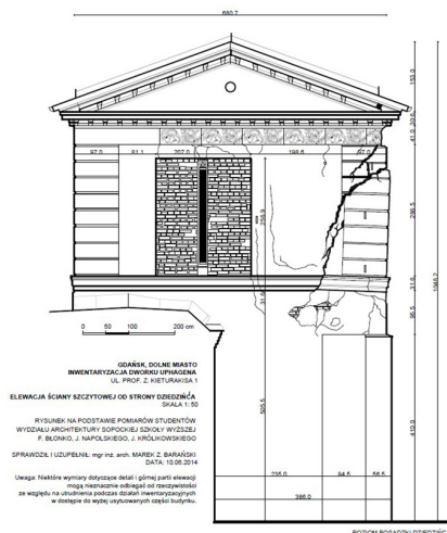
Ryc. 1. Inwentaryzacja elewacji skrzydła dworku Uphagena na Dolnym Mieście w Gdańsku
