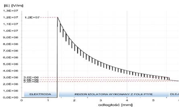
Rys. 6. Wykres natężenia pola elektrycznego w izolatorze w środkowej części – symulacja E – rozkład pola dla szczegółu A
