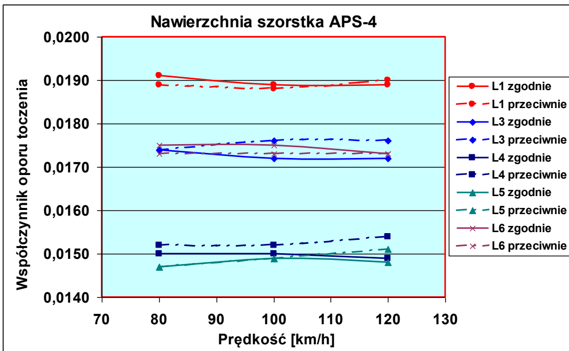
Rysunek 24. Opór toczenia opon kierunkowych z drogową rzeźbą bieżnika, toczonej zgodnie i przeciwie do kierunku oznaczonego na oponie na nawierzchni APS-4 [2]
