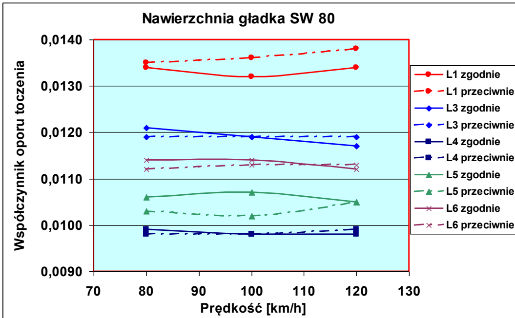
Rysunek 23. Opór toczenia opon kierunkowych z drogową rzeźbą bieżnika, toczonej zgodnie i przeciwie do kierunku oznaczonego na oponie na nawierzchni SW-80 [2]
