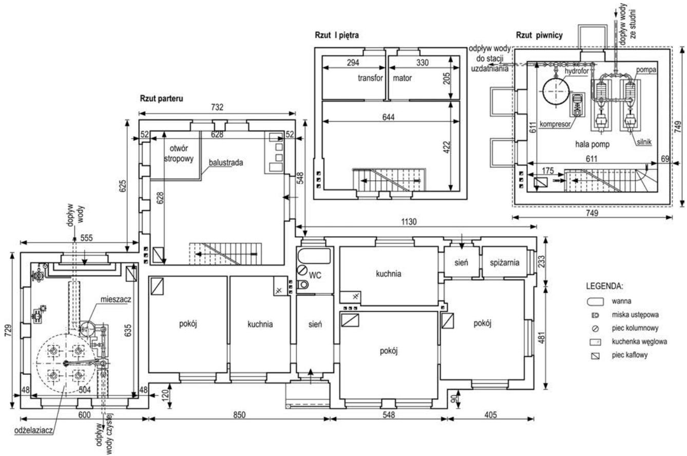
Rys. 3. Rzuty kondygnacji budynku hali pomp, stacji uzdatniania i mieszkań na ujęciu „Oksywie” (opracowanie własne na podstawie materiałów archiwalnych AP Gd. 768/28)
