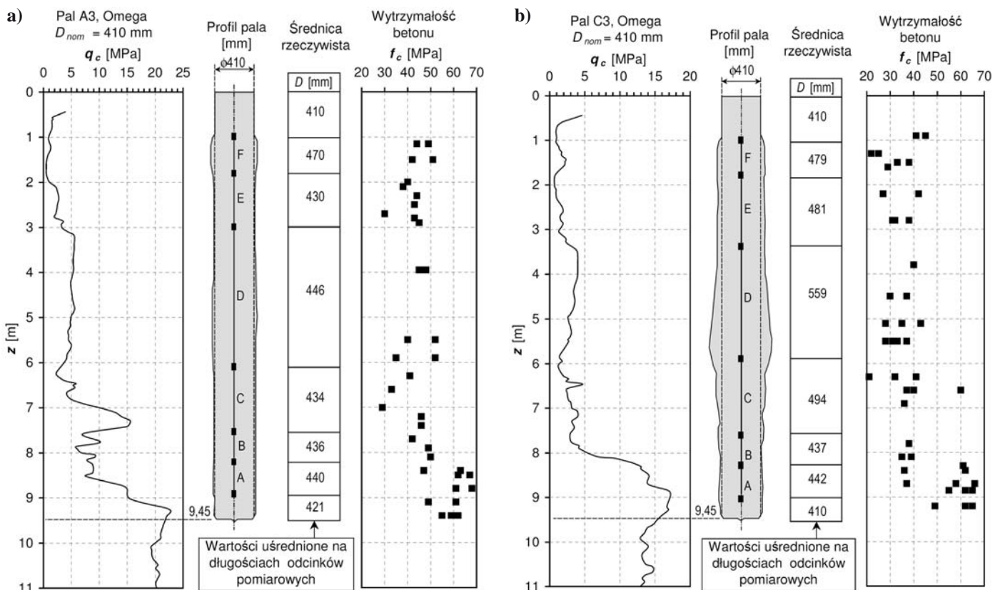
Rys. 3. Przykładowe wyniki badań belgijskich dotyczące niejednorodności przekroju i wytrzymałości betonu w trzonach pali wkręcanych, [3]
