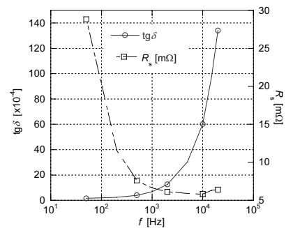
Rys. 4. Charakterystyki \text{tg}\delta i R_S w funkcji częstotliwości f pomierzone dla kondensatora typu MKSP-118 ( 7,5\mu\text{F}/425\text{V} ) przy napięciu skutecznym polaryzacji 1\text{V} ; pomiary wykonano mostkiem RLC GenRad 1689M
