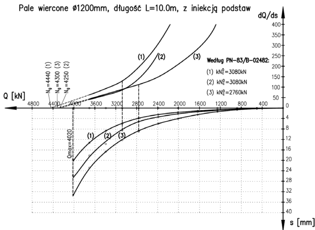
Rys. 4. Wykresy próbných obciążeń pali do przykładu 1
