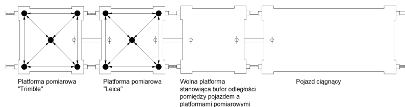
8. Schemat ideowy konstrukcji pomiarowej wykorzystywanej w pomiarach wstępnych
