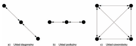
7. Wybrane warianty rozmieszczenia odbiorników GNSS względem osi podłużnej platformy w procesie wyznaczania osi toru
