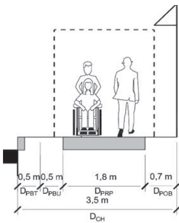
Rys. 17. Przykład minimalnych szerokości chodnika w korytarzach ulic położonych na obszarach intensywnej gęstości zabudowy Źródło: opracowanie własne
