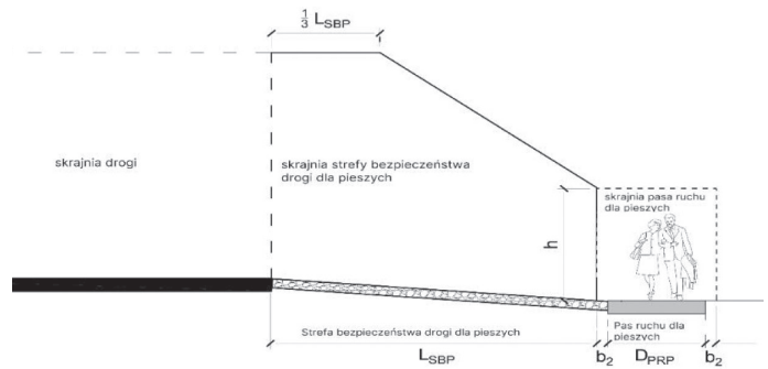
Rys. 11. Usytuowanie drogi dla pieszych wzdłuż drogi zamiejskiej lub ulicy poza strefą bezpieczeństwa drogi Źródło: opracowanie własne
