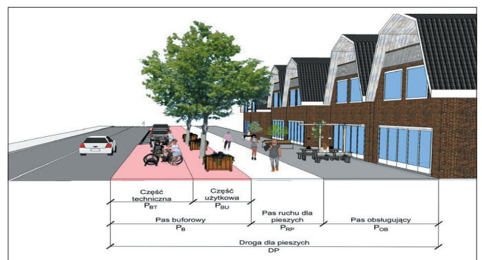
Rys. 9. Schemat podziału przekroju poprzecznego drogi dla pieszych na pasy funkcjonalne
