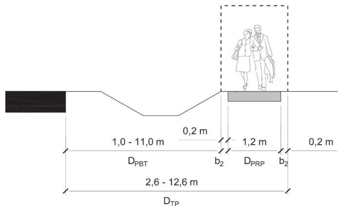
Rys. 19. Przykład minimalnej szerokości ścieżki dla pieszych wraz z pasami funkcjonalnymi, dla ścieżki dla pieszych w korytarzu drogi zamiejskiej Źródło: opracowanie własne
