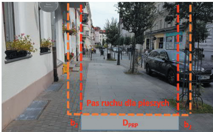
Rys. 20. Pas ruchu dla pieszych – schemat ustalania szerokości, źródło: opracowanie własne
