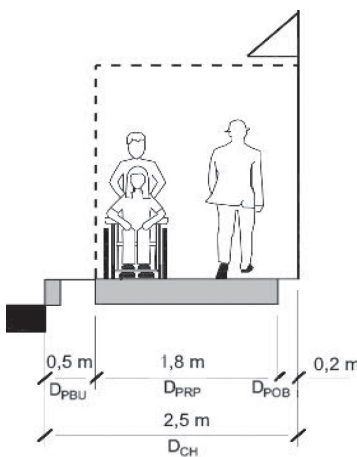
Rys. 18. Przykład minimalnych szerokości chodnika w korytarzach ulic położonych na obszarach ekstensywnej i umiarkowanej gęstości zabudowy Źródło: opracowanie własne
