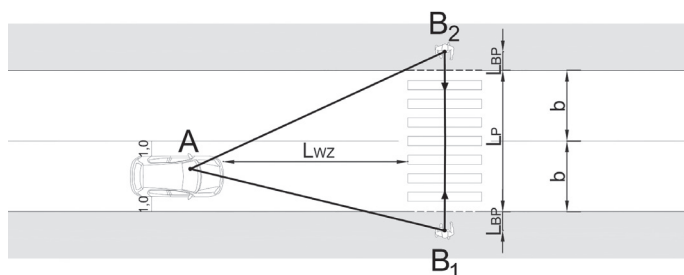
Rys. 12. Pole widoczności pieszego z punktu widzenia kierowcy pojazdu
