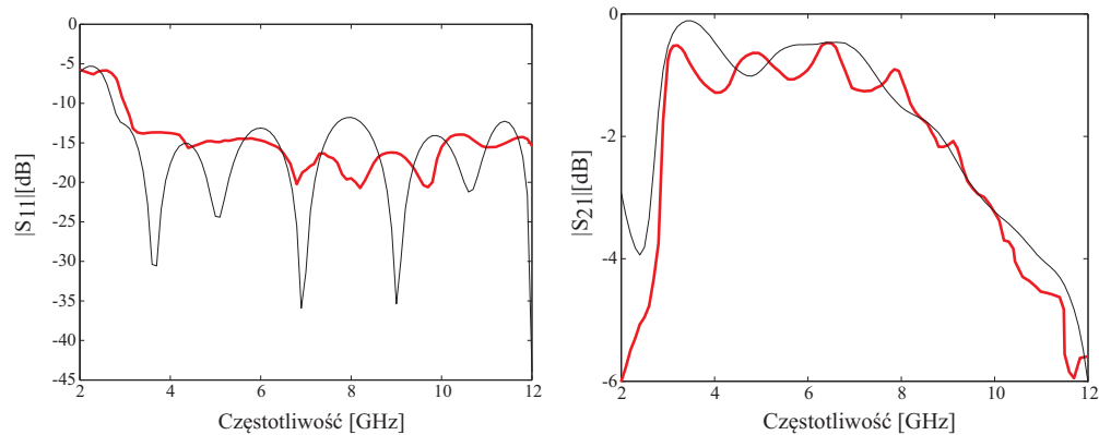
RYSUNEK 6.3: Charakterystyki modułów współczynnika odbicia i transmisji symetryzatora wzorcowego w konfiguracji przeciwsoonej z odcinkiem linii (wynik symulacji - kolor czarny, wynik pomiaru - kolor czerwony)
