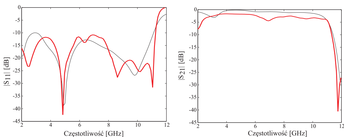
RYSUNEK 6.12: Charakterystyki modułów współczynnika odbicia i transmisji symetryzatora z sękiem prostokątnym zaprojektowanego na podłożu Duroid 6006 w konfiguracji przeciwsobnej przy połączeniu bezpośrednim (wynik symulacji - kolor czarny, wynik pomiaru - kolor czerwony)
