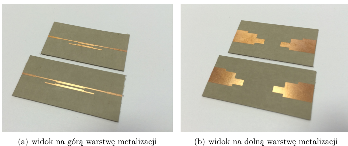
RYSUNEK 6.11: Zdjęcie przedstawiające dwa zrealizowane układy przeciwsobne symetryzatora z sękiem prostokątnym zaprojektowanego na podłożu Duroid 6006
