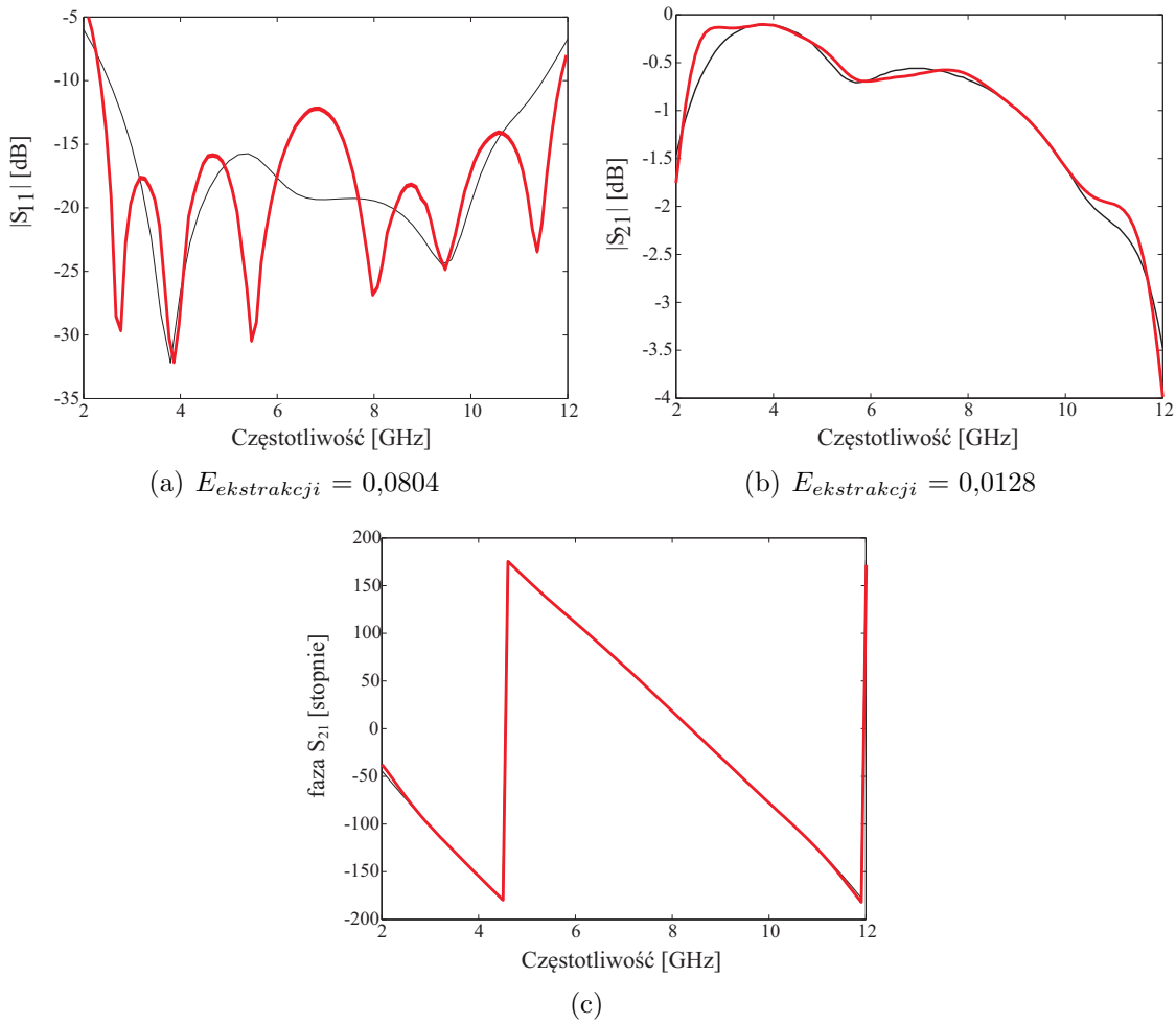
RYСУNEK 5.2: Wyniki ekstrakcji parametrów wzorcowego symetryzatora z sękiem prostokątnym (metoda uproszczona)
