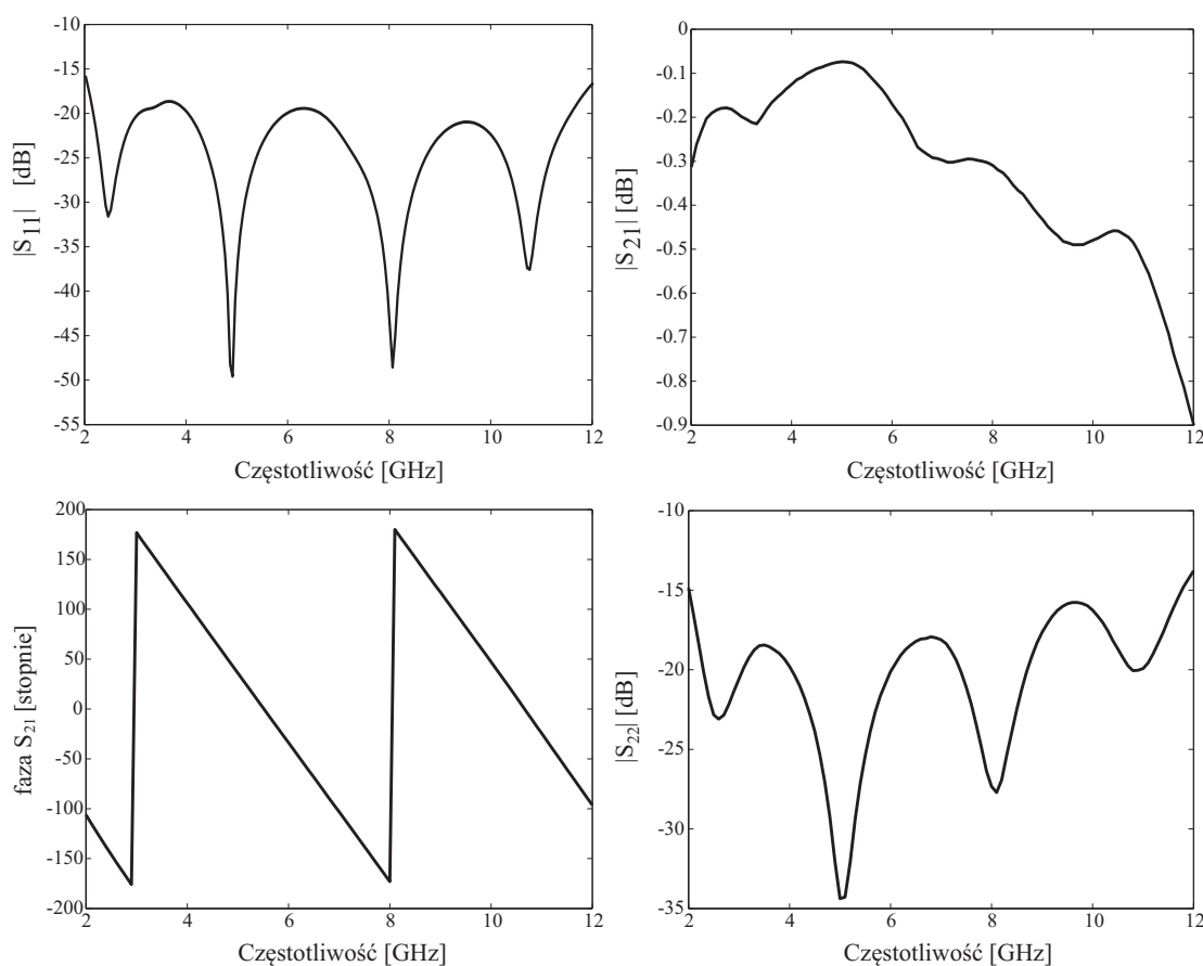
RYСУNEK 4.2: Charakterystyki częstotliwościowe parametrów rozpraszania symetryzatora z rys. 4.1
