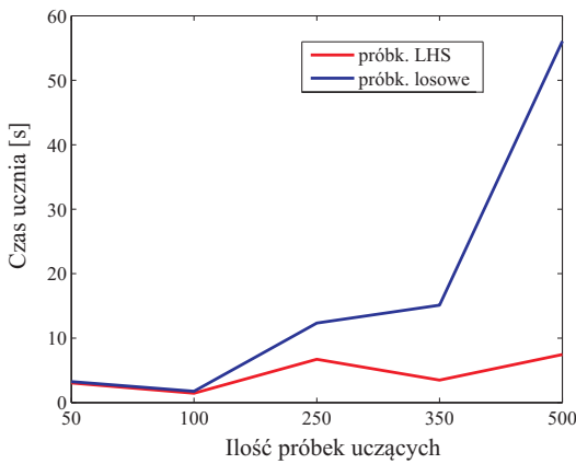
(a) 10 neuronów w warstwie ukrytej
