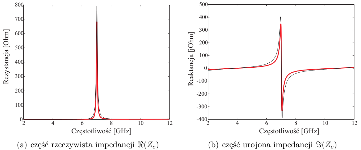
RYSUNEK 2.5: Wyniki modelowania sęka prostokątnego na podłożu Rogers RT Duroid 6006 (czerwony) na tle parametrów sęka wzorcowego (czarny)
