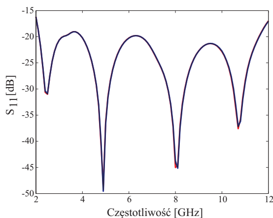
(c) Błąd wymiarów \pm 0,001 ( E_{rms} = 10^{-6} ) \bar{E}_{gen-proj} = 0,00038
