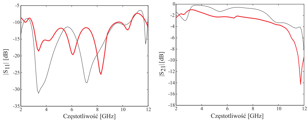
RYSUNEK 6.13: Charakterystyki modułów dopasowania i transmisji symetryzatora z sękiem prostokątnym zaprojektowanego na podłożu Duroid 6006 w konfiguracji przeciwsoonej z odcinkiem linii (wynik symulacji - kolor czarny, wynik pomiaru - kolor czerwony)
