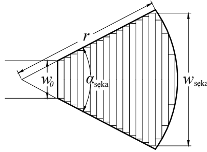
RYSUNEK 2.7: Model numeryczny sęka radialnego ( r - promień sęka, w_{\text{sęka}} - szerokość sęka, \alpha_{\text{sęka}} - kąt rozwarcia sęka, w_0 - szerokość linii zasilającej)
