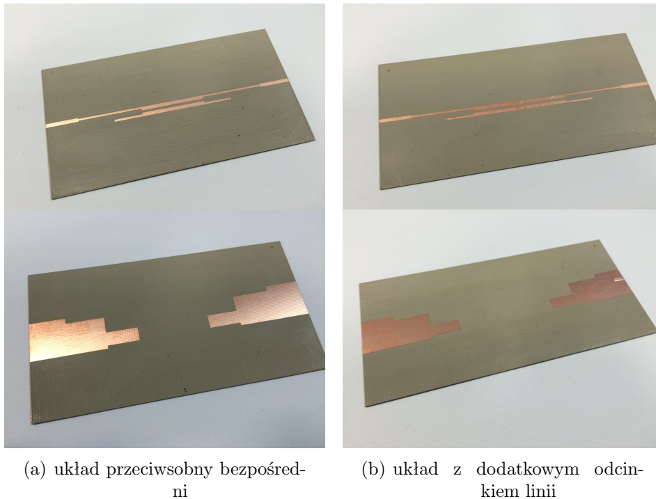
RYSUNEK 6.6: Zdjęcie przedstawiające dwa zrealizowane układy przeciwsobne symetryzatora z sękiem prostokątnym zaprojektowanego na częstotliwość środkową f = 3,5 GHz
