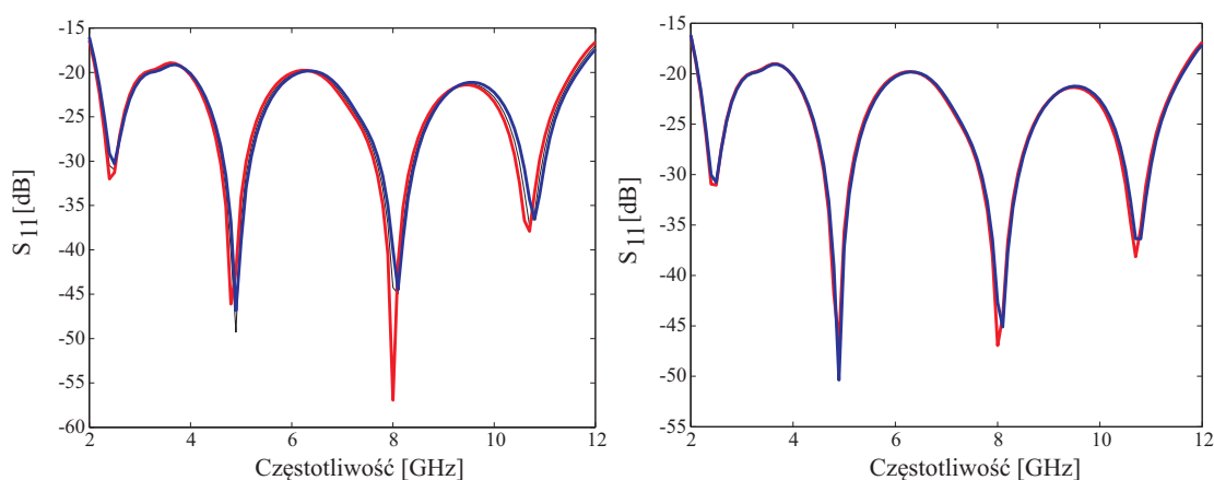
(a) Błąd wymiarów \pm 0,01 ( E_{rms} = 10^{-4} ) \bar{E}_{gen-proj} = 0,0039
