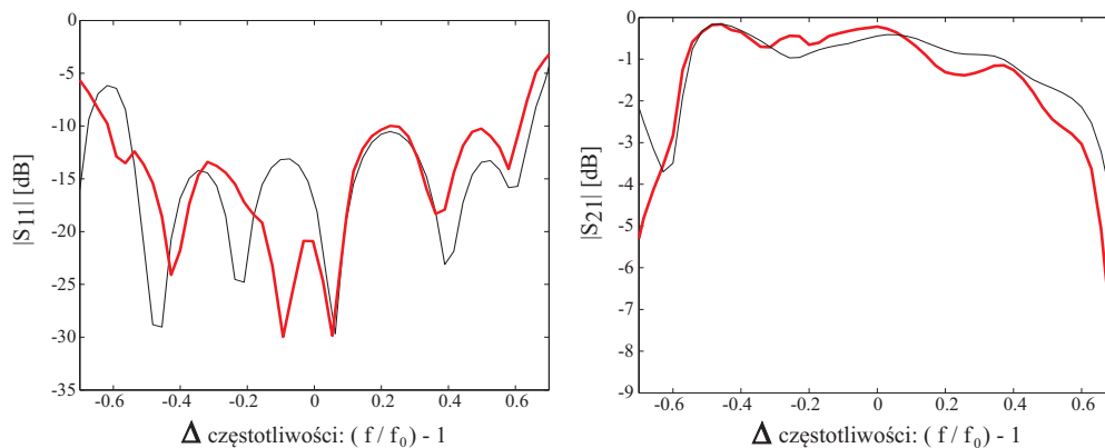
RYSUNEK 6.7: Charakterystyki modułów współczynnika odbicia i transmisji symetryzatora z sękiem prostokątnym zaprojektowanego na częstotliwość środkową f = 3,5 GHz w konfiguracji przeciwsobnej przy, połączeniu bezpośrednim - rys. 6.6(a) (wynik symulacji - kolor czarny, wynik pomiaru - kolor czerwony)
