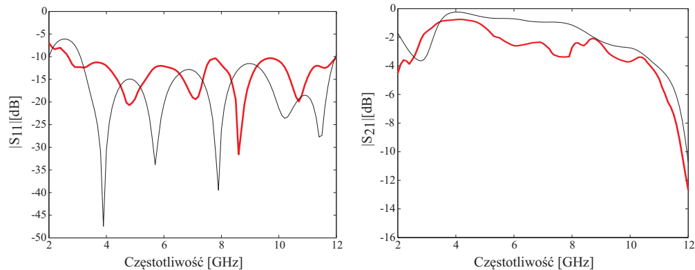
RYSUNEK 6.2: Charakterystyki modułów współczynnika odbicia i transmisji symetryzatora wzorcowego w konfiguracji przeciwsoonej przy połączeniu bezpośrednim (wynik symulacji - kolor czarny, wynik pomiaru - kolor czerwony)
