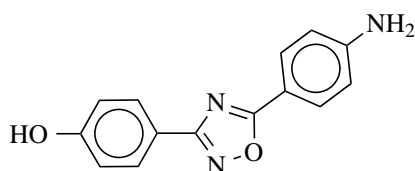
4-(5-(4-Aminofenylo)-1,2,4-oksadiazol-3-ilo)fenol 37
