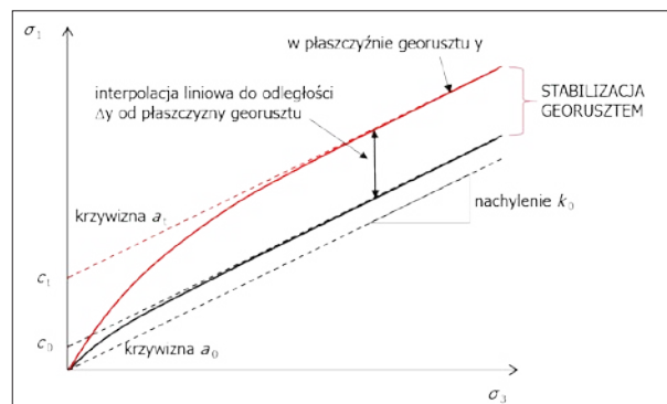
Rys. 3. Graniczny stan naprężenia kruszywa stabilizowanego georusztem heksagonalnym [12]
