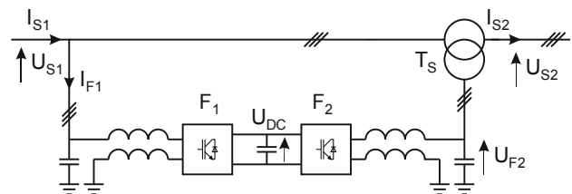
Rys. 3. Energoelektroniczny regulator napięcia
