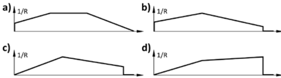
3. Wykresy stosowanych krzywizn w torach zwrotnych rozjazdów klotoidalnych [8, 10]
