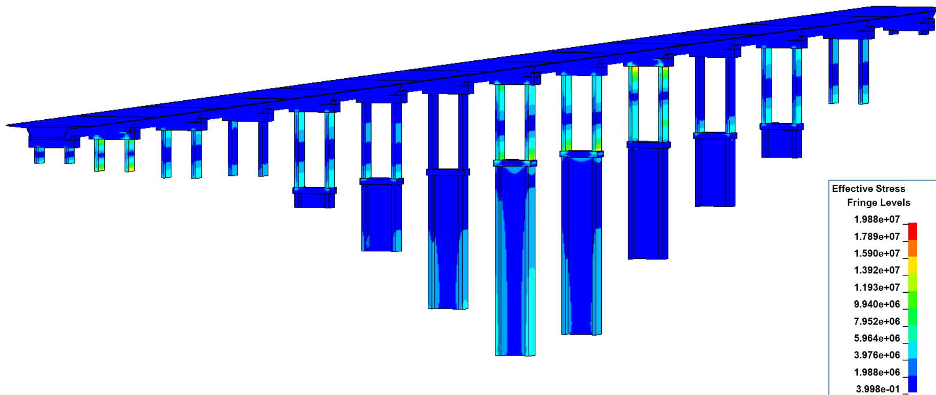
Rys. 133 Analiza zniszczeń wiaduku V17 - według rozwiązania autorskiego - stan wiaduku po czasie t=100 [s] trwania trzęsienia ziemi Kocaeli z poziomu D1
