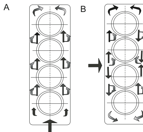
Rys. 2. Schemat wzdłużnego A i poprzecznego B przepływu cieczy chłodzącej przez blok cylindrów załamane strzałki symbolizują odpływ cieczy w kierunku głowicy Fig. 2. In line A and perpendicular B coolant flow through engine block. Broken arrow indicate flow direction engine head
