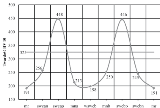
Rys. 14. Rozkład twardości wzdłuż linii A-A (rys. 13) na płycie próbnej ze stali S355J2G3. Poziomą linią zaznaczono HVmax strefy odpuszczanej w SWC pierwszej napoiny (swca2p)
