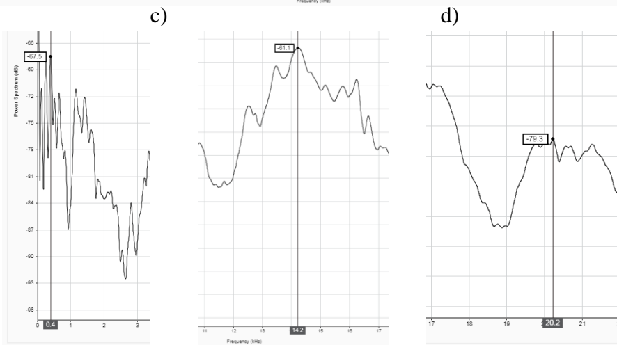
Rys. 12 Widok widma sygnału przyspieszenia drgań - lokalizacja I, oś X; a) pełne widmo w zakresie 0 – 25 kHz; b), c), d) – powiększone fragmenty widma
