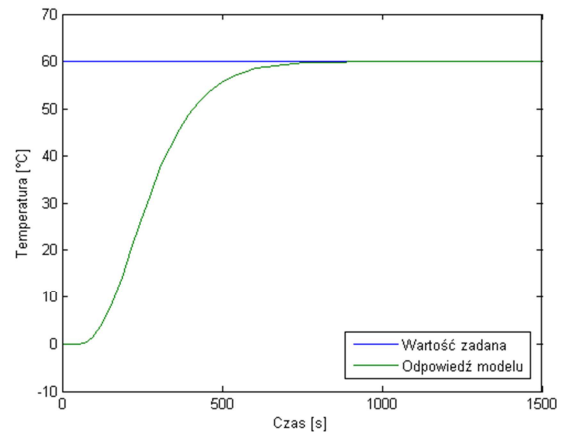
Rys. 19. Odpowiedź układu (model z 4 zmiennymi stanu)
