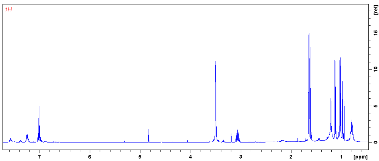
Widmo 11. Widmo ^1\text{H} kryształów kompleksu [\text{Me}_6\text{NacNacTi}(\text{Cl})\{\eta^2\text{-P-P}(\text{Ph})\text{tBu}\}] ( 2C ) rozpuszczonych w \text{C}_6\text{D}_6 .
