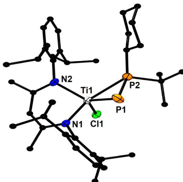
Rys. 31. Struktura kompleksu [ Me NacNacTi(Cl){η 2 -P-P(Cy)tBu}] ( 5B ), wybrane długości wiązań (Å) i miary kątów (°): N1-Ti1 2,046(3), N2-Ti1 2,034(3), P1-P2 2,1039(19), P1-Ti1 2,3153(15), P2-Ti1 2,5079(16), Cl1-Ti1 2,3059(13); P1-P2-Ti1 59,50(5), N1-Ti1-N2 93,30(14), P1-Ti1-P2 51,54(5). Suma kątów wokół atomu fosforu ΣP2 = 330,2.
