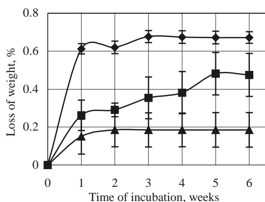
Fig. 6. Weight loss of PEUR after incubation in hydrogen peroxide solution: ■ — PEUR-1, ▲ — PEUR-2, ◆ — PEUR-3
