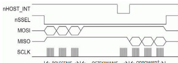
Rys. 5. Procedura komunikacji między modułem ZigBee i hostem
