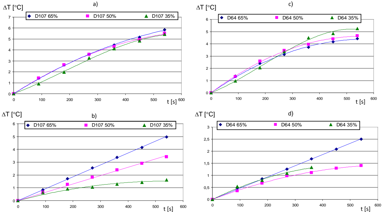
Rys. 6. Przyrost temperatury PO ( \text{Al}_2\text{O}_3 ) podczas szlifowania ściernicami o spoiwie galwanicznym z ziarnami diamentowymi bez zużycia początkowego CPS: a) D107, c) D64 oraz ze zużyciem początkowym CPS: b) D107, d) D64
