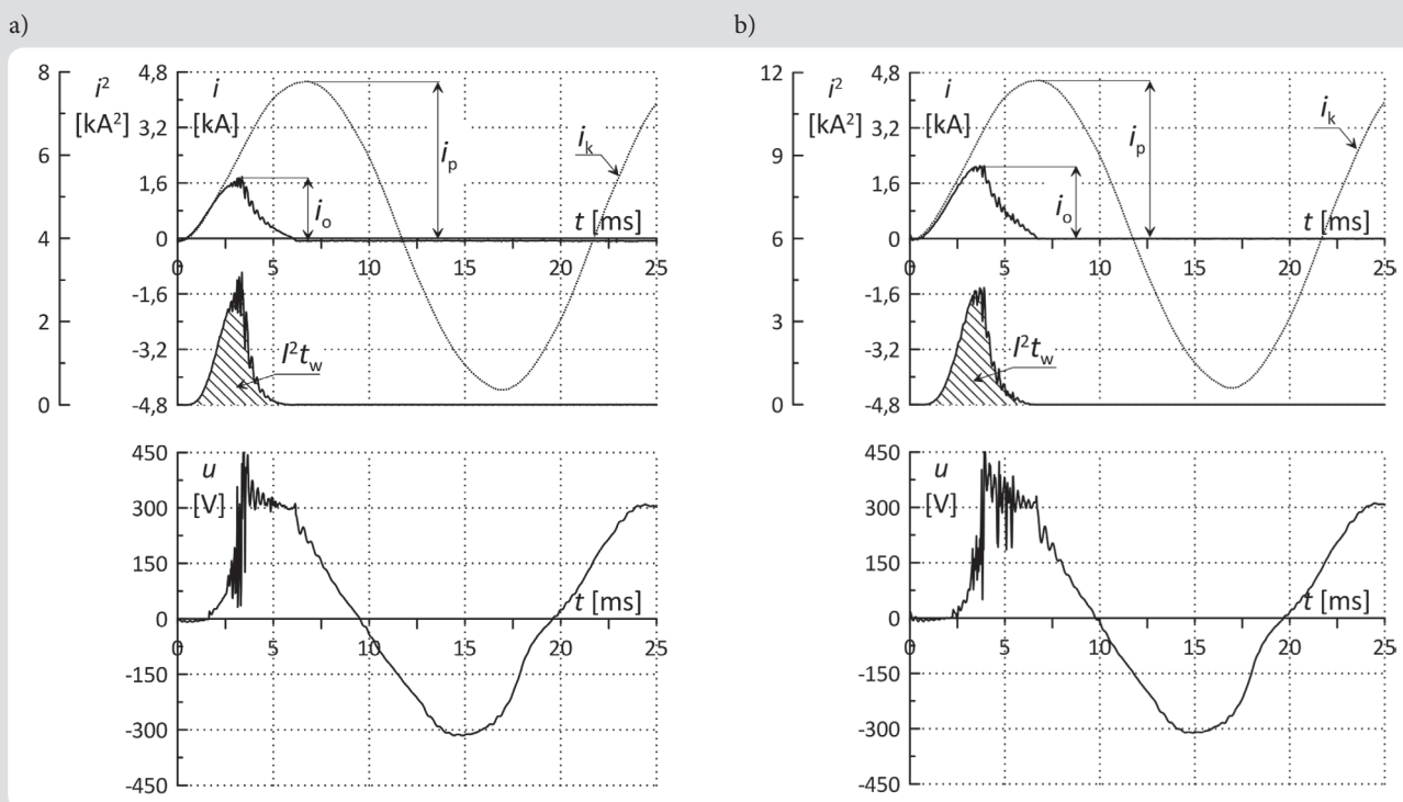
Rys. 3. Wyłączenie prądu zwarcia przez wyłącznik nadprądowy instalacyjny; I_k = 3,1 kA, i_p = 4,5 kA, a) wyłącznik C16, i_0 = 1,8 kA, P^2 t_w = 4,8 kA 2 s, b) wyłącznik D20, i_0 = 2,1 kA, P^2 t_w = 7,9 kA 2 s
