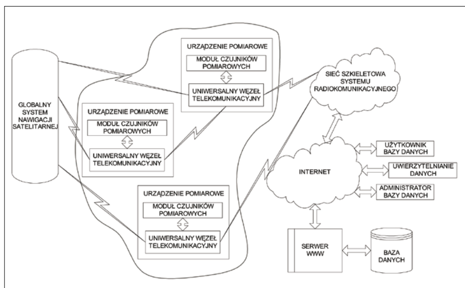
Rys. 1. Schemat funkcjonalny bezprzewodowego systemu monitorowania zagrożeń bezpieczeństwa
