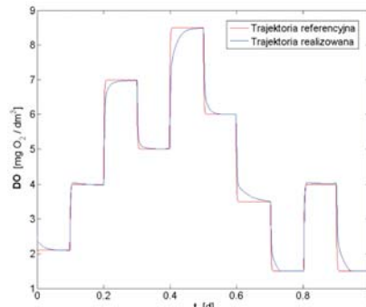
Rys. 9. Wartość zadana i zrealizowana stężenia tlenu w komorze tlenowej
