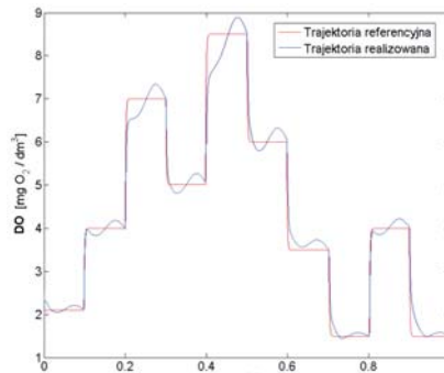
Rys. 12. Wartość zadana i zrealizowana stężenia tlenu w komorze tlenowej
