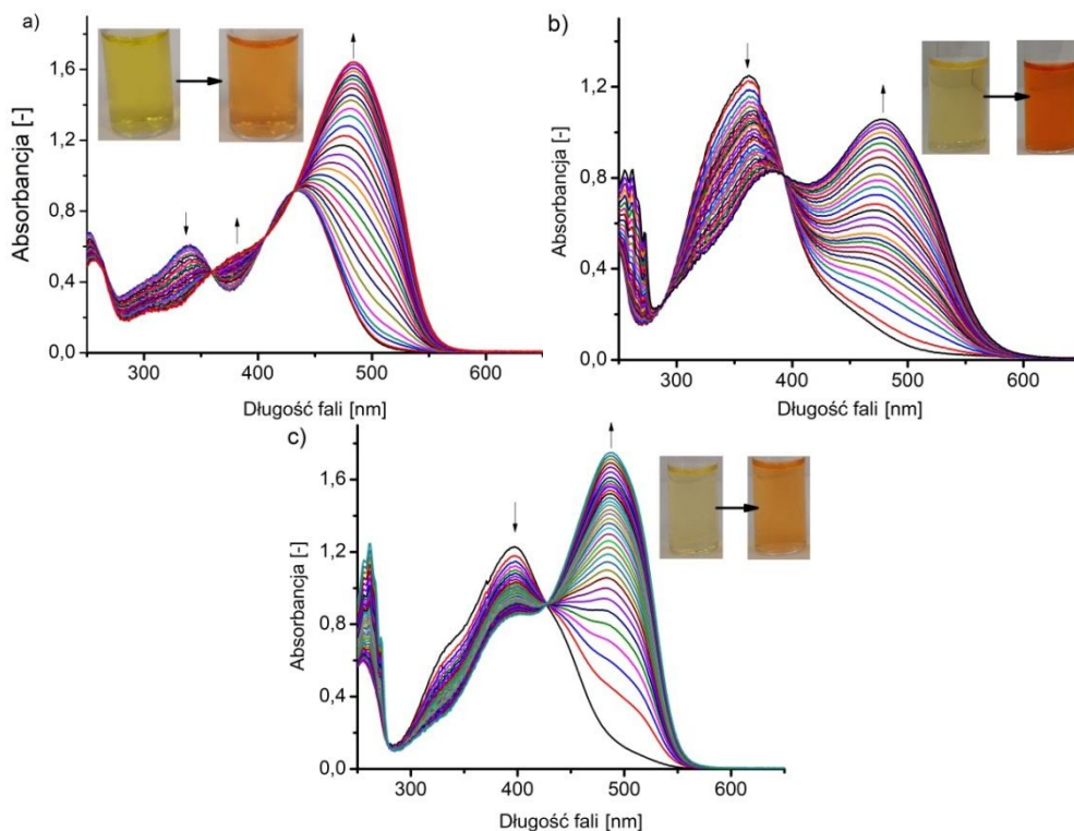
Rys. 4.14. Zmiany w widmie absorpcyjnym podczas miareczkowania kwasem para -toluenosulfonowym (TosOH) oraz zmiana barwy roztworu hydroksyazobenzokoron w obecności kwasu dla: a) związku 19-p-OH ( c = 5,6 \cdot 10^{-5} \text{ mol/dm}^3 ); c_{\text{TosOH}} = 0-9,1 \cdot 10^{-5} \text{ mol/dm}^3 , b) związku 19-o-OH ( c = 7,6 \cdot 10^{-5} \text{ mol/dm}^3 ); c_{\text{TosOH}} = 0-7,6 \cdot 10^{-5} \text{ mol/dm}^3 , c) związku 21-o'-OH ( c = 7,4 \cdot 10^{-3} \text{ mol/dm}^3 ); c_{\text{TosOH}} = 0-1,4 \cdot 10^{-3} \text{ mol/dm}^3 w acetonitrylu
