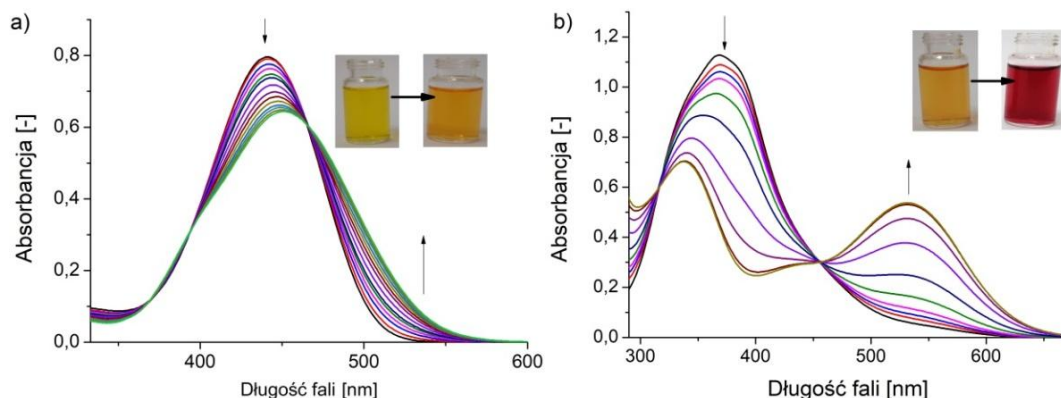
Rys. 4.19. Zmiany w widmie absorpcyjnym podczas miareczkowania roztworem wodorotlenku tetra-n -butyloamoniowego (TBAOH) a) związku t-Bu-19-p-OH ( c = 2,09 \cdot 10^{-5} \text{ mol/dm}^3 ); c_{\text{TBAOH}} = 0 - 8,14 \cdot 10^{-5} \text{ mol/dm}^3 , b) związku t-Bu-19-o-OH ( c = 6,96 \cdot 10^{-5} \text{ mol/dm}^3 ); c_{\text{TBAOH}} = 0 - 1,38 \cdot 10^{-3} \text{ mol/dm}^3 w acetonitrylu
