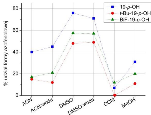
Rys. 4.10. Procentowy udział formy azofenolowej badanych para -hydroksyazobenzokoron: 19- p -OH , t -Bu-19- p -OH oraz BiF-19- p -OH (stężenie \sim 10^{-5} mol/dm 3 ) w zależności od rozpuszczalnika wyznaczony na podstawie widm absorpcyjnych
