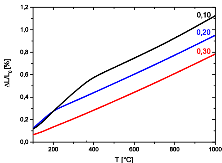
Rysunek 6.12 Wydłużenie względne próbek LaNb_{1-x}Sb_xO_4 w funkcji temperatury. 170
