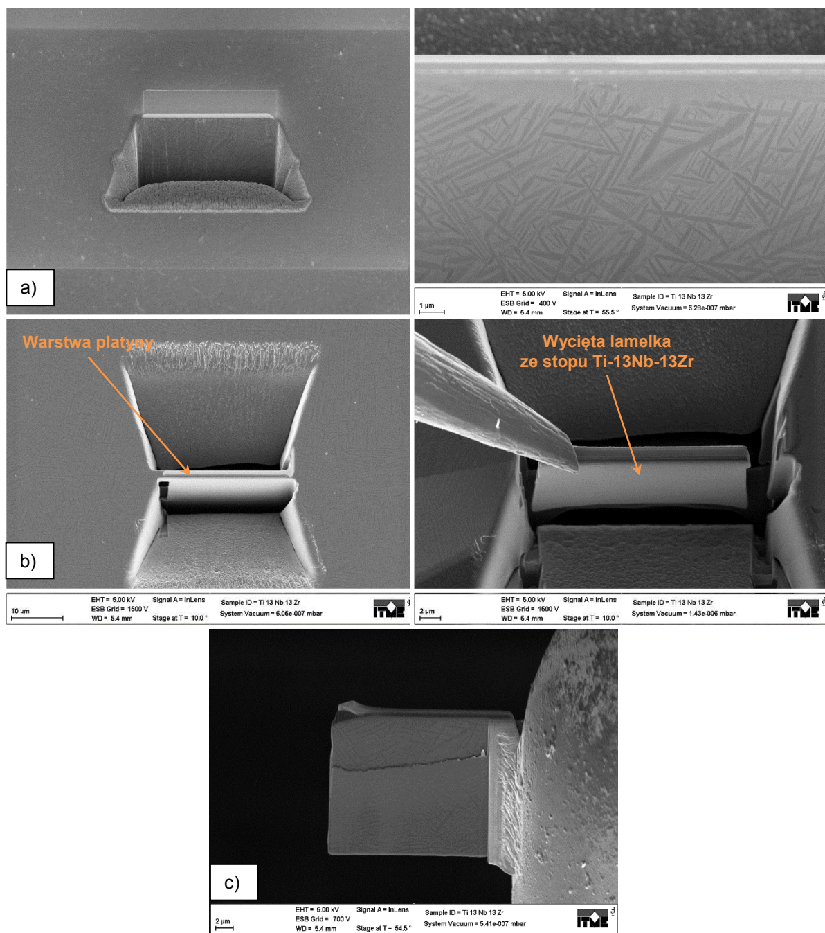
Rys. 53. Etapy przygotowania lamelki ze stopu Ti-13Nb-13Zr z wykorzystaniem metody FIB (Focused ion beam): a) wytypowany obszar do badań pokryty warstwą platyny, b) wycinanie lamelki oraz przeniesienie jej z materiału rodzimego na siateczkę za pomocą igły, c) pocienianie lamelki
