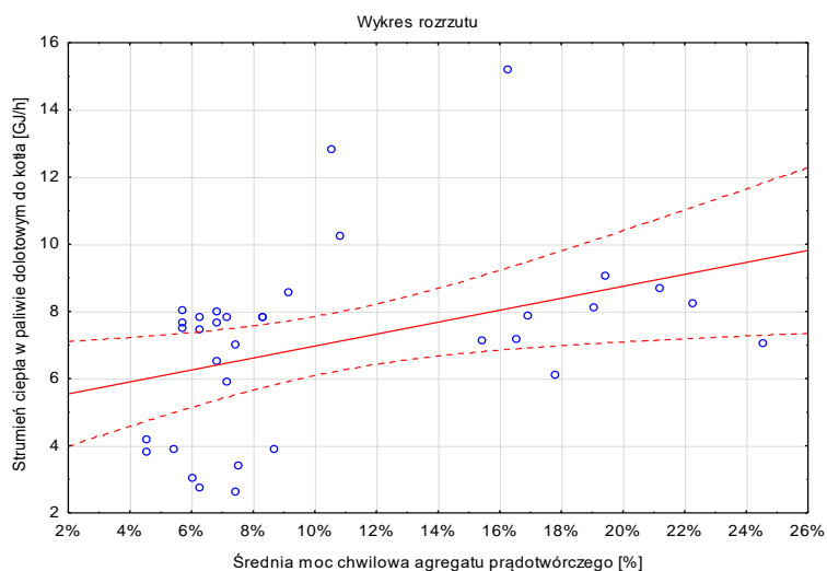
Rys. 4 Wykres korelacji strumienia ciepła dolotowego do kotła a średniej mocy chwilowej agregatów prądowórczych
