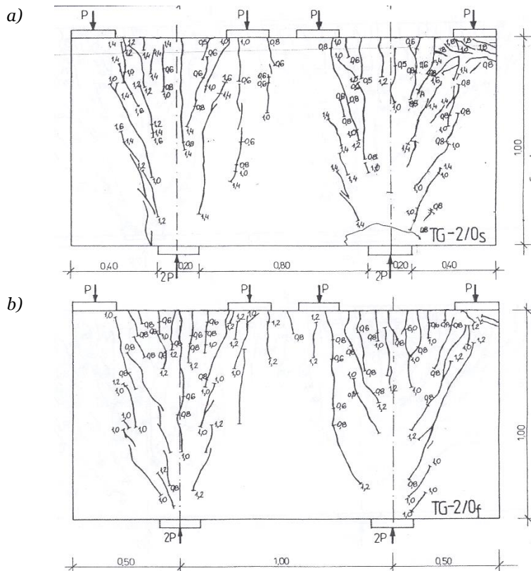
Rys. 3.16 Morfologia rys tarcz TG-2 zbrojonych ortogonalnie [7]: a) tarcza TG-2/Os, b) tarcza TG-2/Of [11].
