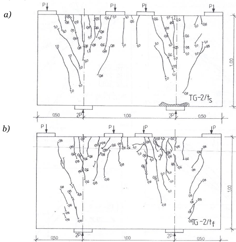
Rys. 3.17 Morfologia rys tarcz TG-2 zbrojonych trajektorialnie [7]: a) tarcza TG-2/ts, b) tarcza TG-2/tf [11].
