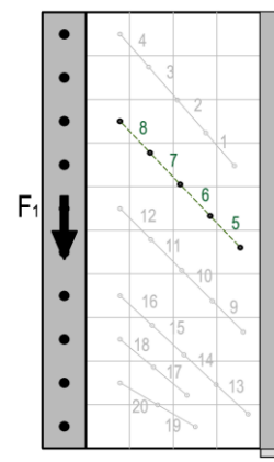
Rys. 4.49 Odształcenia betonu na kierunku ściskanego krzyżulca (nr bazy 5-8) tarczy wspornikowej układu DB II-0.5.
