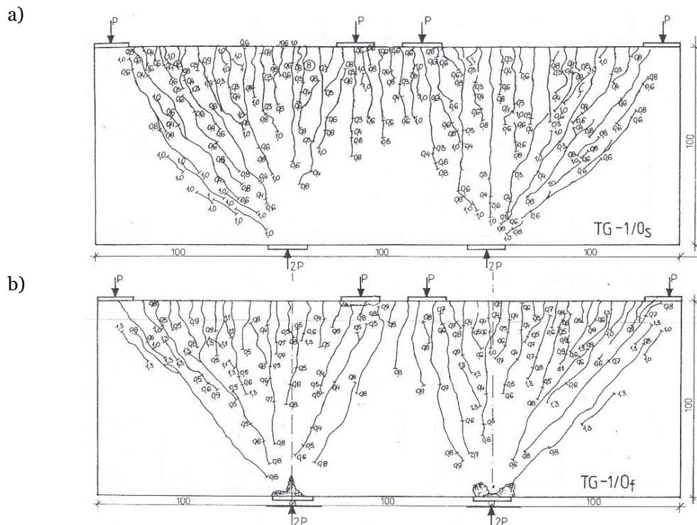
Rys. 3.14 Morfologia rys tarcz TG-1 zbrojonych ortogonalnie [7]: a) tarcza TG-1/0 s , b) tarcza TG-1/0 f [11].
