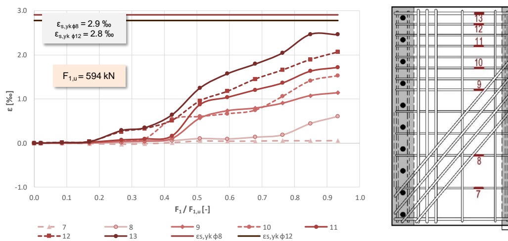
Rys. 4.34 Odkształcenia stali zbrojenia poziomego tarczy wspornikowej układu DB II-0.5 .
