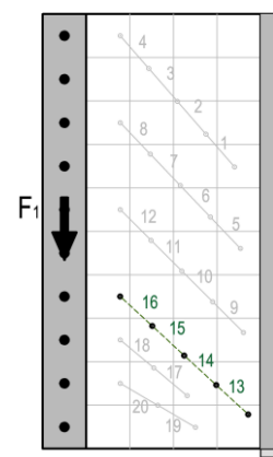
Rys. 4.51 Odształcenia betonu na kierunku ściskanego krzyżulca (nr bazy 13-16) tarczy wspornikowej układu DB II-0.5.
