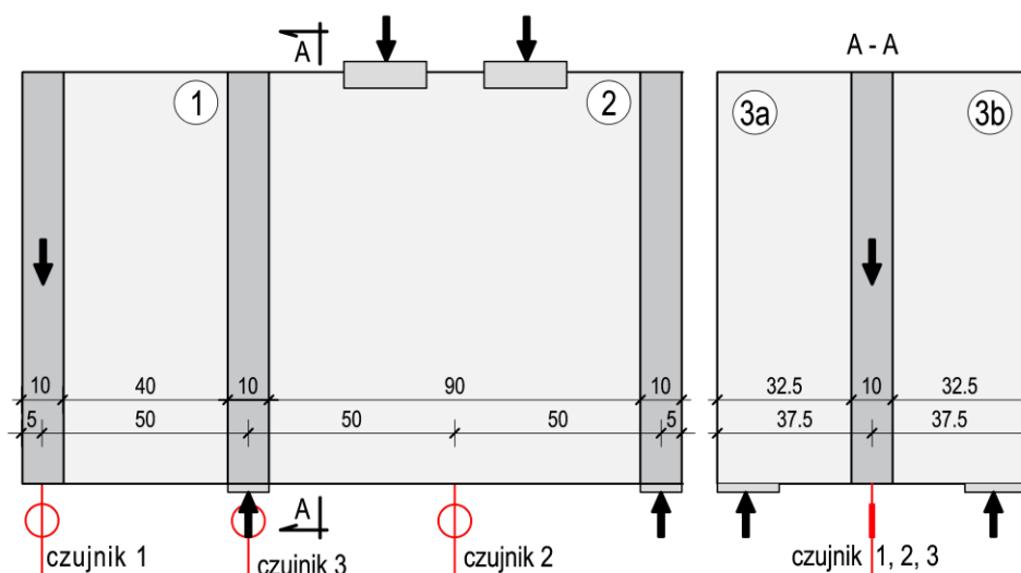
Rys. 4.26 Rozmieszczenie czujników indukcyjnych dla tarcz układu DB-0.5 (I seria).
