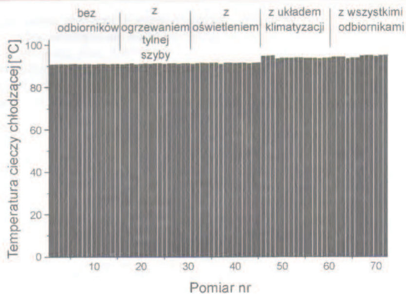
Rys. 7. Średnie temperatury cieczy chłodzącej podczas wszystkich pomiarów w testach EPA4X. Fig. 7. Mean Coolant temperatures during all EPA4X tests.
