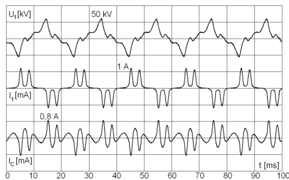
Rys. 4. Zarejestrowane przebiegi prądu I_1 w uzwojeniu pierwotnym przekładnika średniego napięcia (1 A/dz.), prądu I_C w pojemności rezonanowej (0,8 A/dz.) oraz napięcia U_1 na uzwojeniu pierwotnym w warunkach ferorezonansu (50 kV/dz.)
