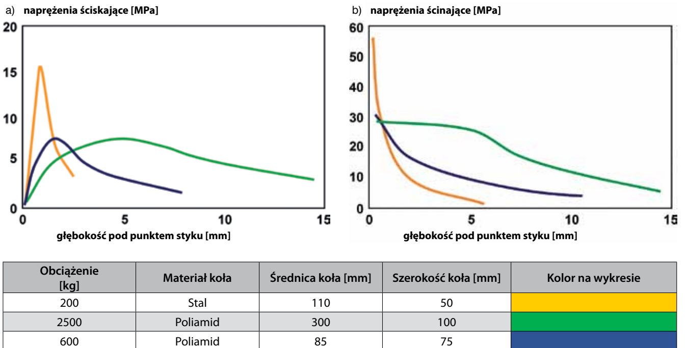
Rys. 2. Naprężenia: a) ściskające, b) ścinające na posadzce betonowej w zależności od rodzaju ogumienia pojazdów, według [34]
