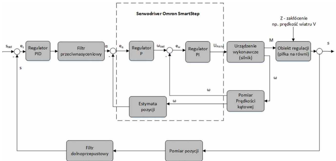
Rys. 10. Schemat blokowy układu regulacji
