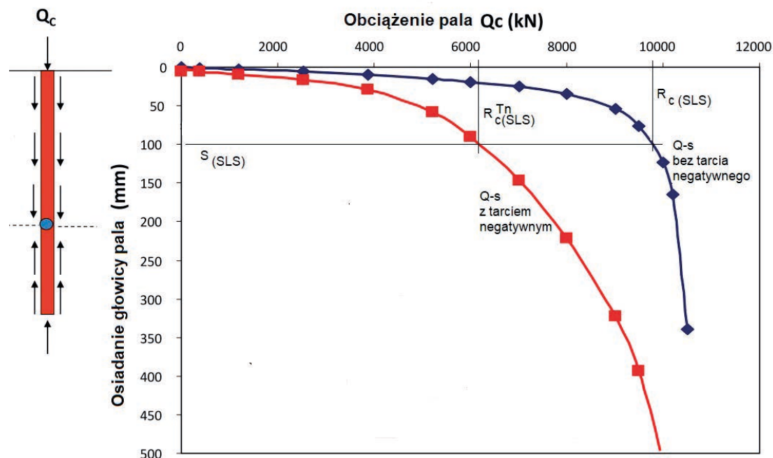
Rys. 5. Przykładowe próbnego obciążenie pala o średnicy 1,0 m z tarcieniem negatywnym i bez tarcia negatywnego [6]
