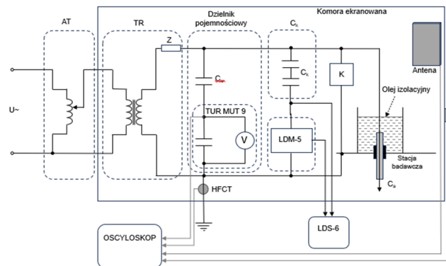
Rys.2 Schemat układu probierczego do badania izolatorów przepustowych SN, Legenda: U~ - napięcie zasilające, AT - autotransformatorem, TR - transformator probierczy ( S_n = 2,5 kVA, U_{1n}/U_{2n} = 230 V/50 kV, 50 Hz), Z - filtr, C_w - kondensator wzorcowy ( U_n = 55 kV, C_n = 60 pF, p = 0,4 MPa), TUR MUT 9 - przyrząd do pomiaru napięcia, C_k - kondensator sprzęgający ( C_n = 2 \times 1000 pF \pm 10\% , 25 kV, 50 Hz), LDM-5 - impedancja pomiarowa, K - kalibrator LDC-5, C_a - obiekt badany, (HFCT, CC-TEV, Antena) - sondy pomiarowe, LDS-6 - rejestrator wzn firmy Doble, Oscyloskop - TDS5034B firmy Tektronix.
