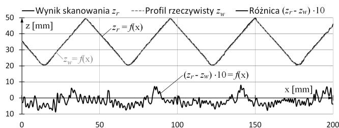
Rys. 8. Wynik skanowania obiektu o dokładnie znanym kształcie i wymiarach
