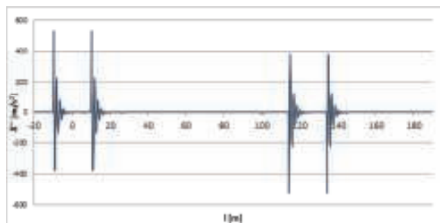
3. Wykresy przyspieszeń ruchu drgającego \ddot{X}(l) dla Przypadku 2 (odcinki krzywizny liniowej, k_1 = k_3 = 1/8000 rad/m)
