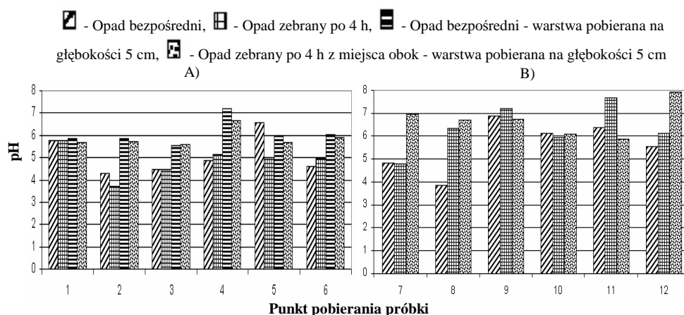
Rys. 7. Wartości pH próbek śniegu zebranych dnia 20.01.2004 w punktach pobierania próbek 1-12 zlokalizowanych: A) na osiedlu Morena w Gdańsku B) na terenie miasta Sopot
