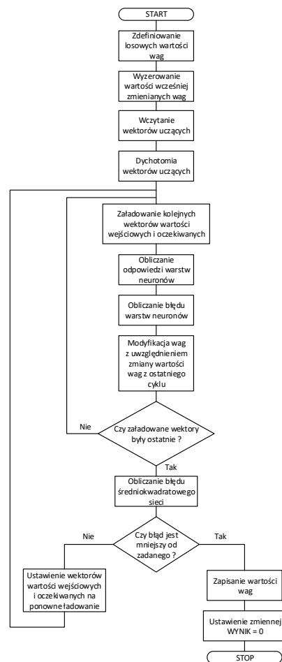
Rys. 6. Algorytm uczenia
