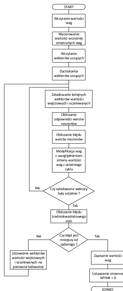
Rys. 7. Algorytm douczania
